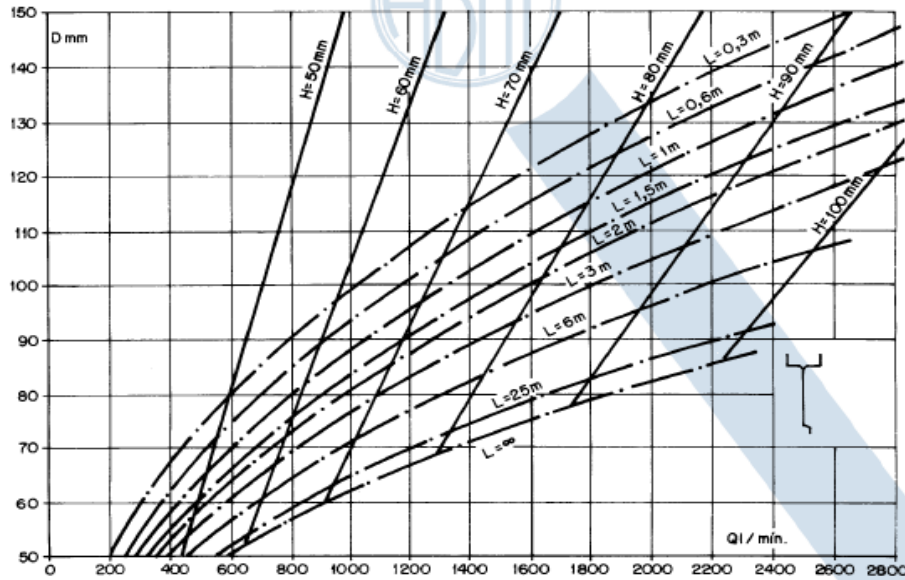
(b) Calha com funil de saída Figura 3 - Ábacos para a determinação de diâmetros de condutores verticais
